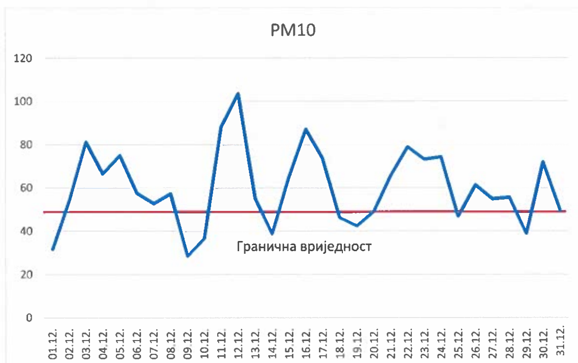
Дијаграм број 8: Графички приказ концентрација РМ10, изражене у µg/m³
