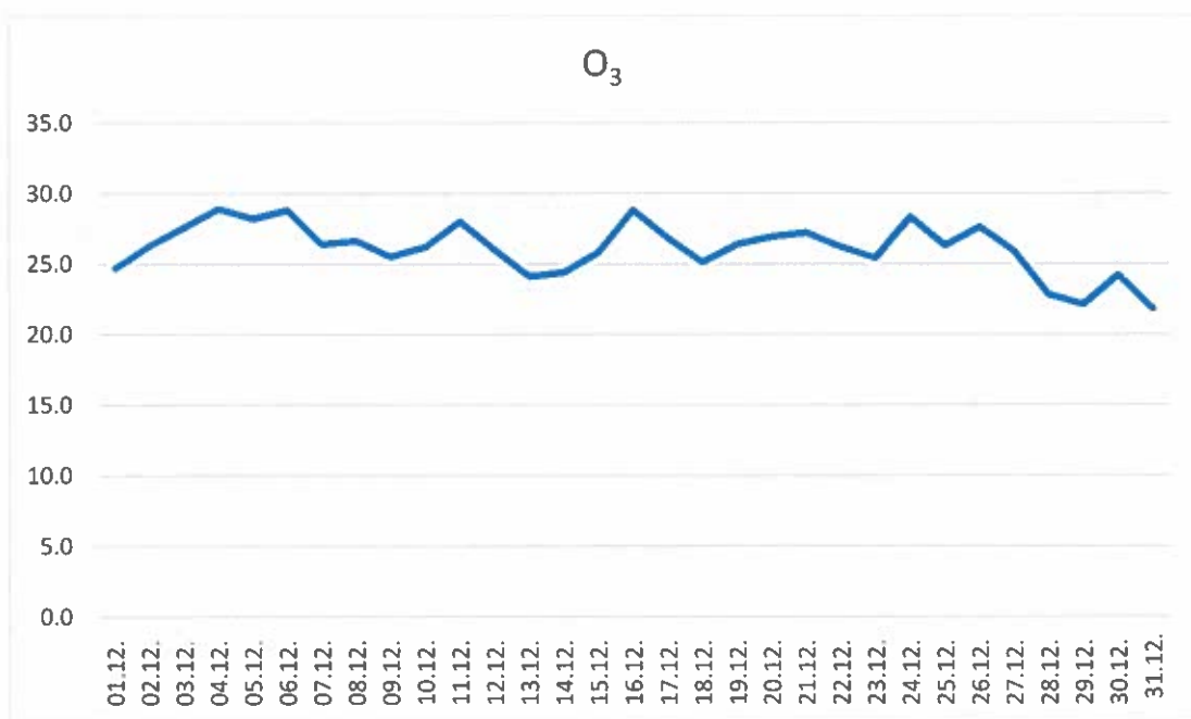
Дијаграм број 6: Графички приказ концентрација озона, изражене у \mu\text{g}/\text{m}^3
