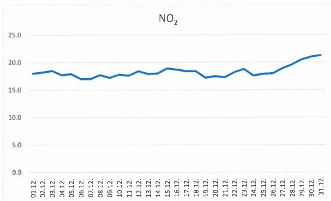
Дијаграм број 3: Графички приказ концентрација азот-диоксида, изражене у µg/m³
