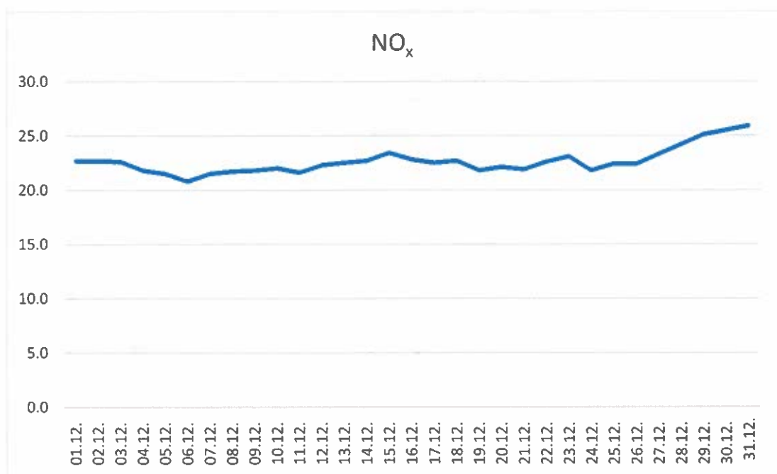
Дијаграм број 5: Графички приказ концентрација азотних оксида, изражене у \mu\text{g}/\text{m}^3
