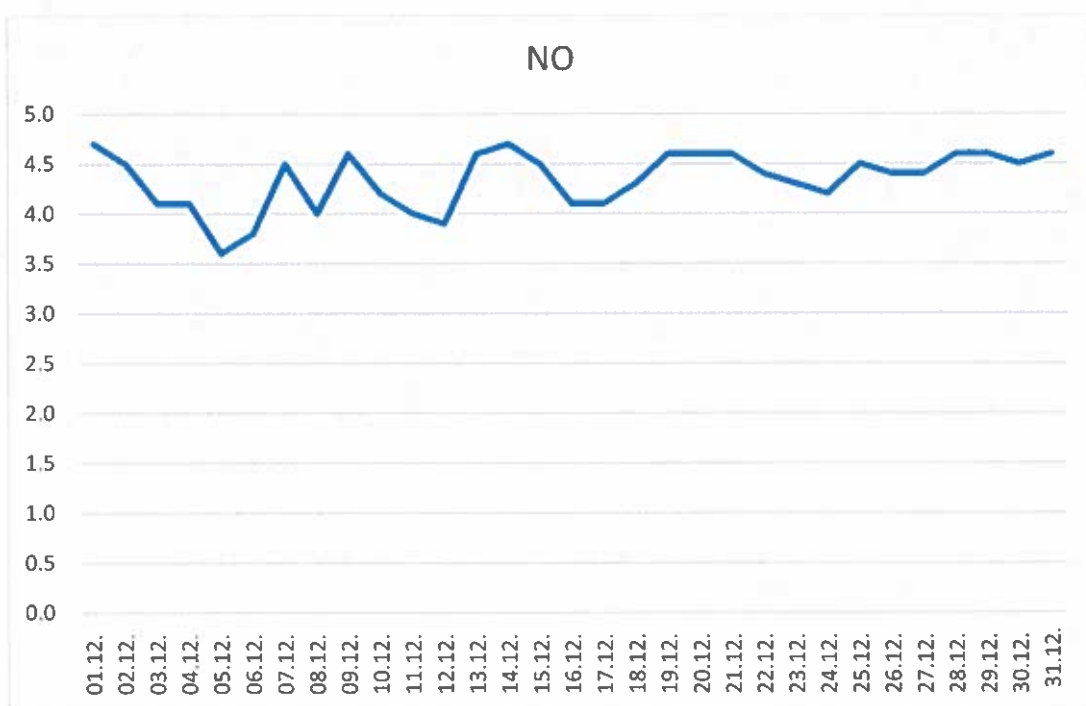
Дијаграм број 4: Графички приказ концентрација азот-монооксида, изражене у µg/m³
